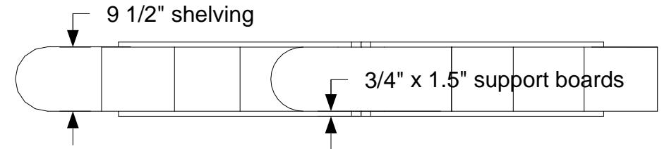
TOP SCALE 1 : 20
